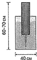
АНКЕРИРАНЕ НА НОСЕЩИТЕ ТРУПИ
